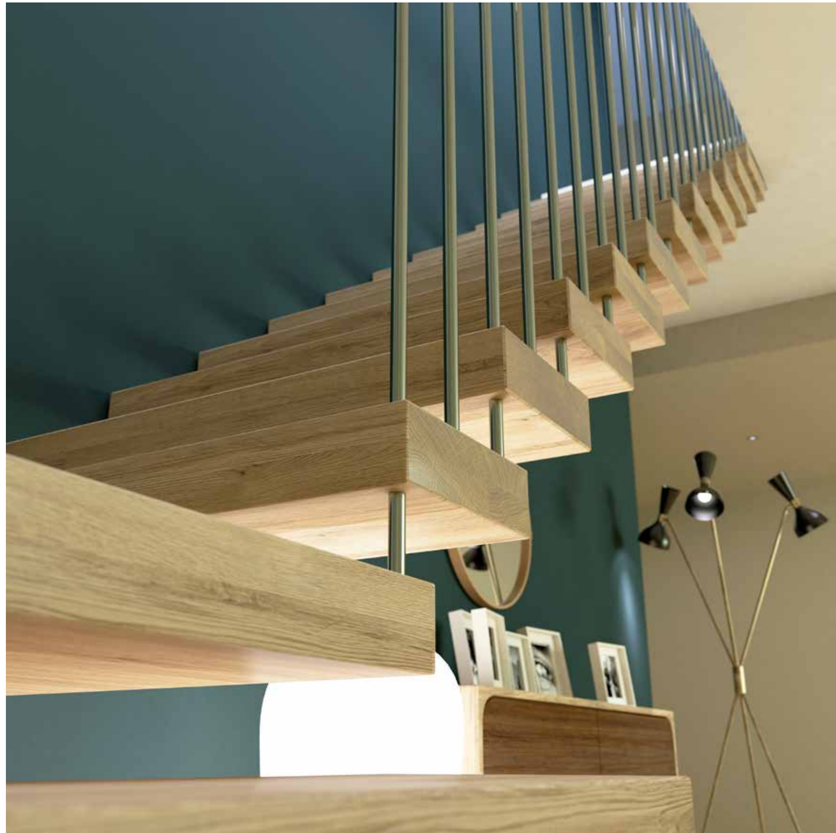
22 Scala a sbalzo con gradini in massello di rovere e tiranti in acciaio inox con diametro di 18 mm. Cantilever staircase with solid oak steps and stainless-steel tension rods with a diameter of 18 mm. Escalier autoportant avec marches en rouvre massif et tirants en acier inox avec diamètre de 18 mm. Kragstufentreppe mit Stufen aus massivem Eichenholz und Zugstangen aus rostfreiem Stahl mit einem Durchmesser von 18 mm. Escalera en voladizo con peldaños de roble macizo y tirantes de acero inoxidable de 18 mm de diámetro.
